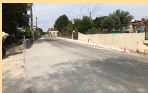
Pousaflôres - Execução de passeio e berma na Estrada dos Peregrinos, São João de Brito
