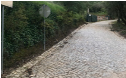
Reparação de Calçada: Freguesia de Ansião - Acesso ao Sr. do Bonfim
